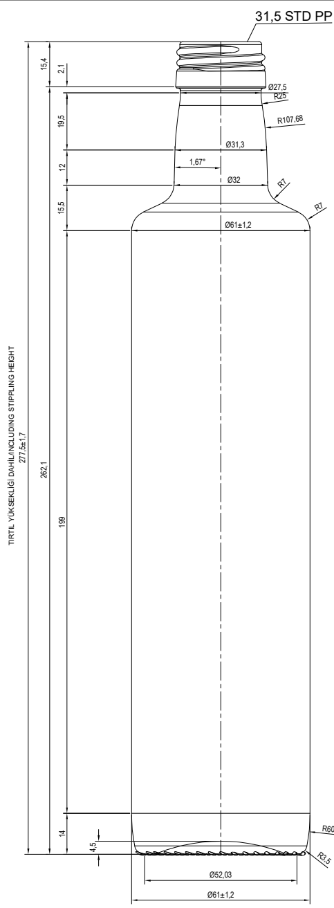
Front view Scale: 1:1
