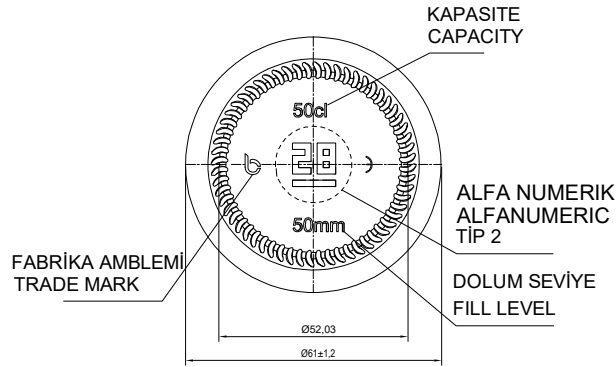
Bottom view Scale: 1:1
