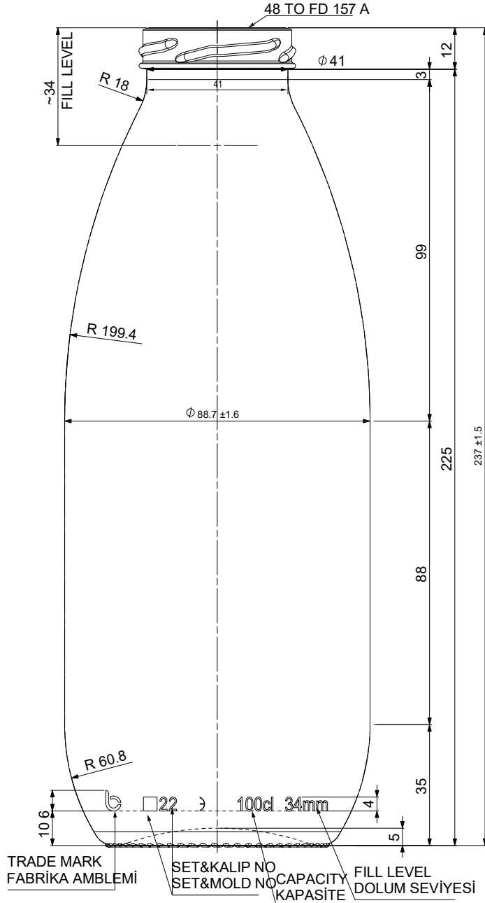
Front view Scale: 1:1
