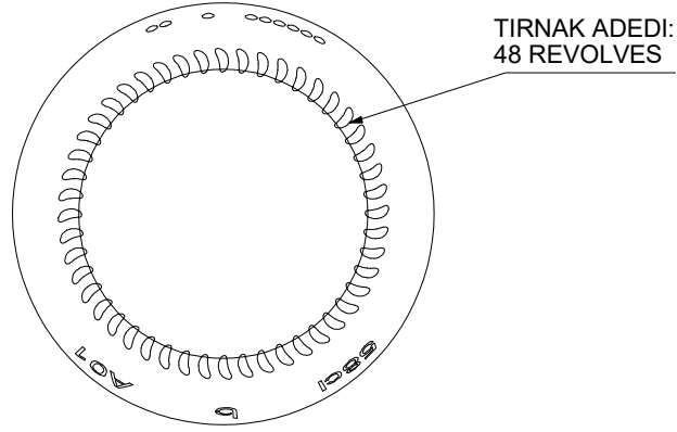
Bottom view Scale: 1:1
