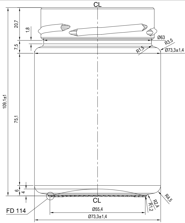
Front view Scale: 1:1
