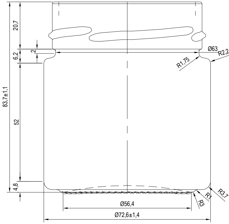
Front view Scale: 1:1
